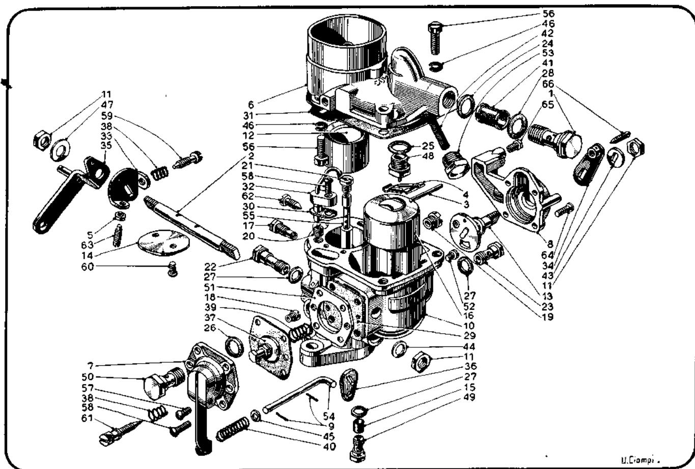
Fig. 01/30 - Carburatore per motori 2" e 3" serie (Dal Catalogo parti di ricambio).
