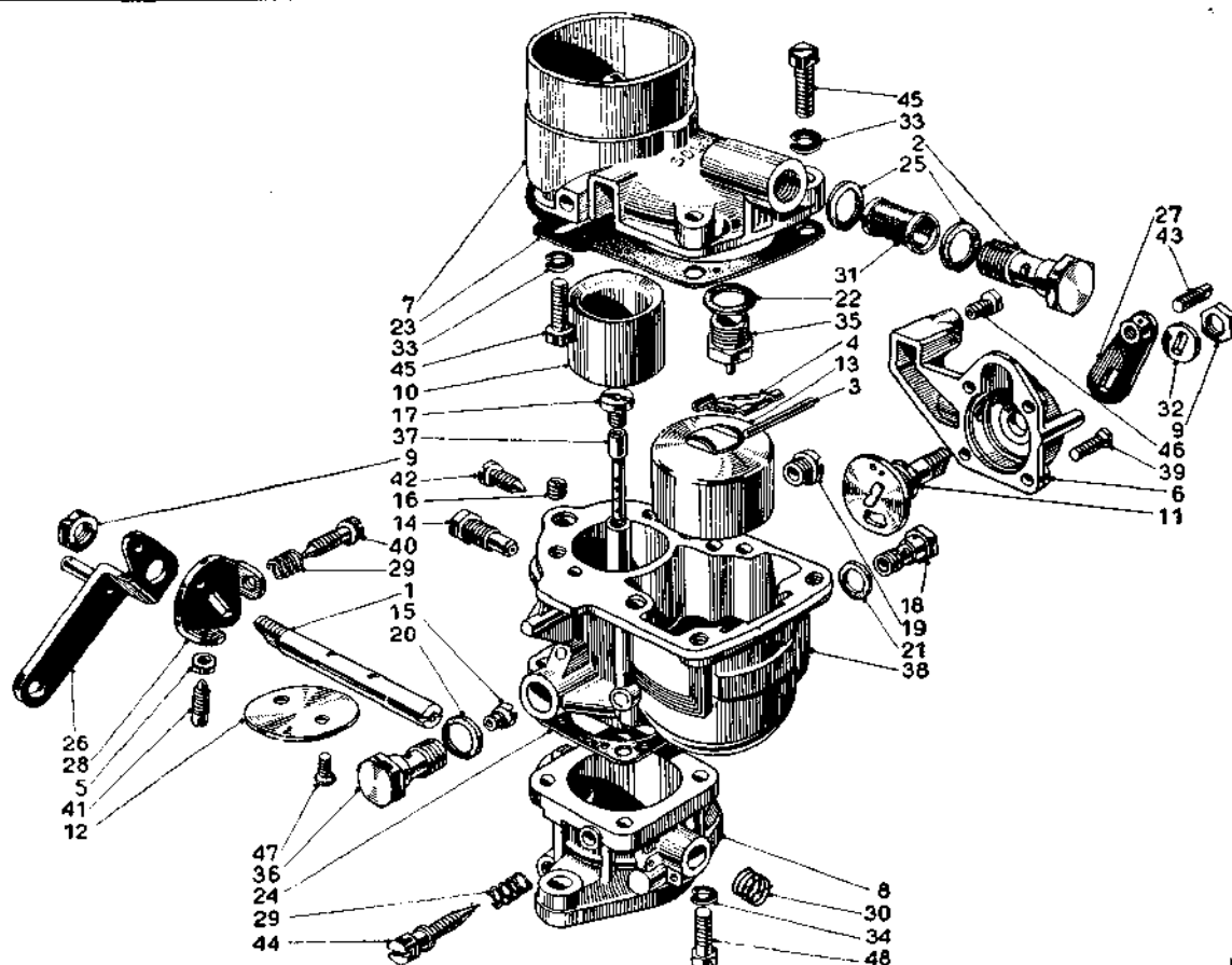
Fig. 01/29 - Carburatore motore 1ª serie (Dal Catalogo parti di ricambio).
