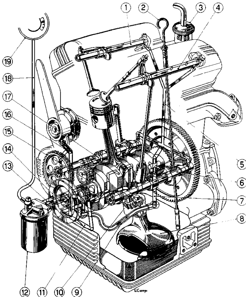
Fig. 01/32 - Lubrificazione motore
