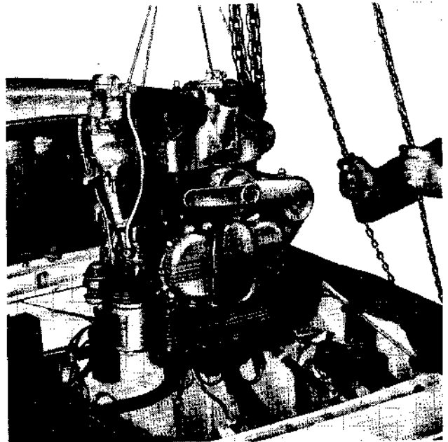
Fig. 01/20 - Sollevamento motore.
