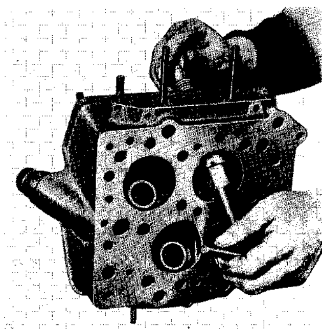
Fig. 01/26 - Ripassatura alloggiamento sedi valvole.
