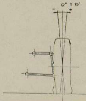
SCHEMA ASSETTO RUOTE SCHEMA ARRANGEMENT DES ROUES
